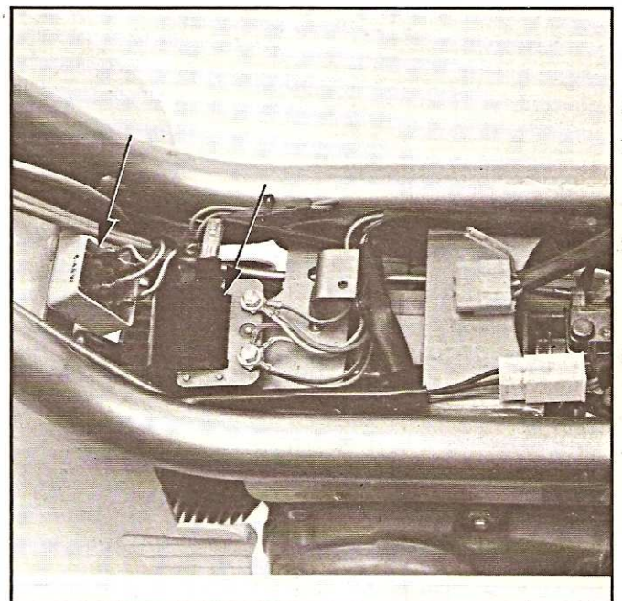
Transformateur 6-4,6 W Bobine H.T. Fig. 24
