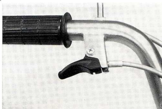
Fig. 46. — JEU DU LEVIER DE DECOMPRESSION.
