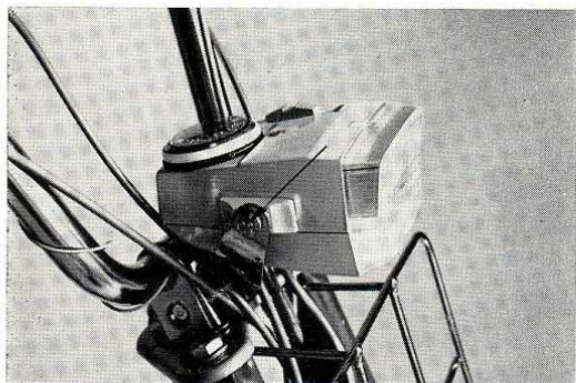
Fig. 3. — DÉMONTAGE DU BOITIER DU PHARE.
