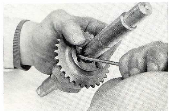
Fig. 80. — DÉMONTAGE DE L'AXE DE PÉDALE.
