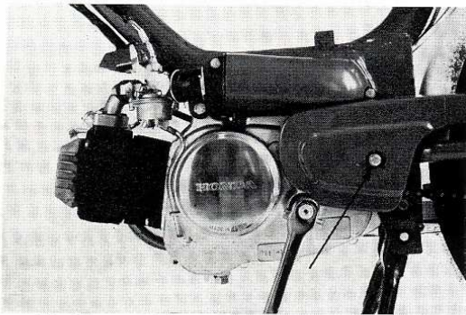
FIG. 27b. — DEMONTAGE DU GARDE-CHAINE.
