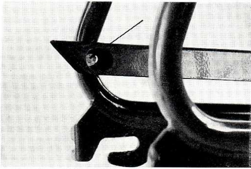
Fig. 27a. — DEMONTAGE DU GARDE-CHAINE.
