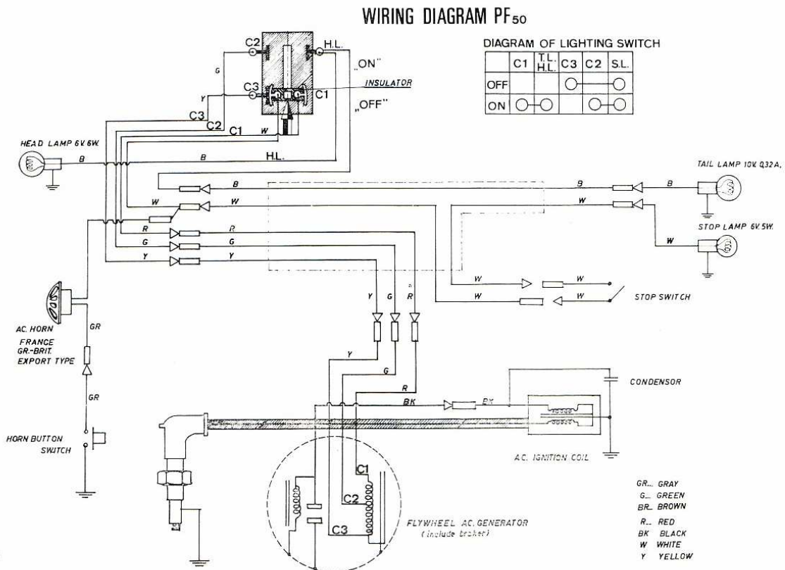
Fig. 37. — Schéma de l'installation électrique.
