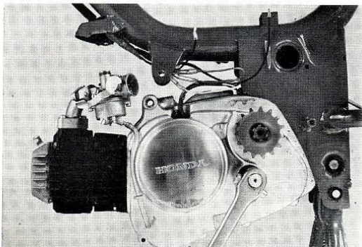
Fig. 29. — DEPOSE DU MOTEUR.
