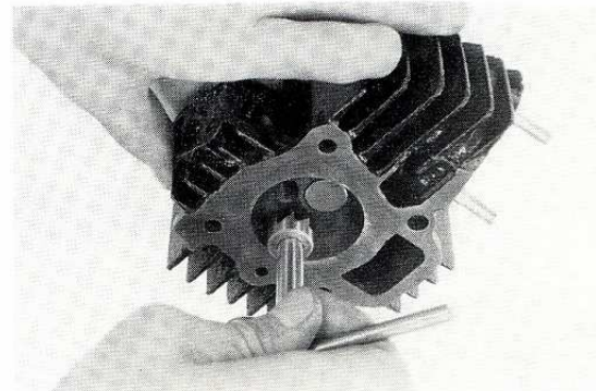
Fig. 58. — REPARATION DU SIEGE DE SOUPE.
