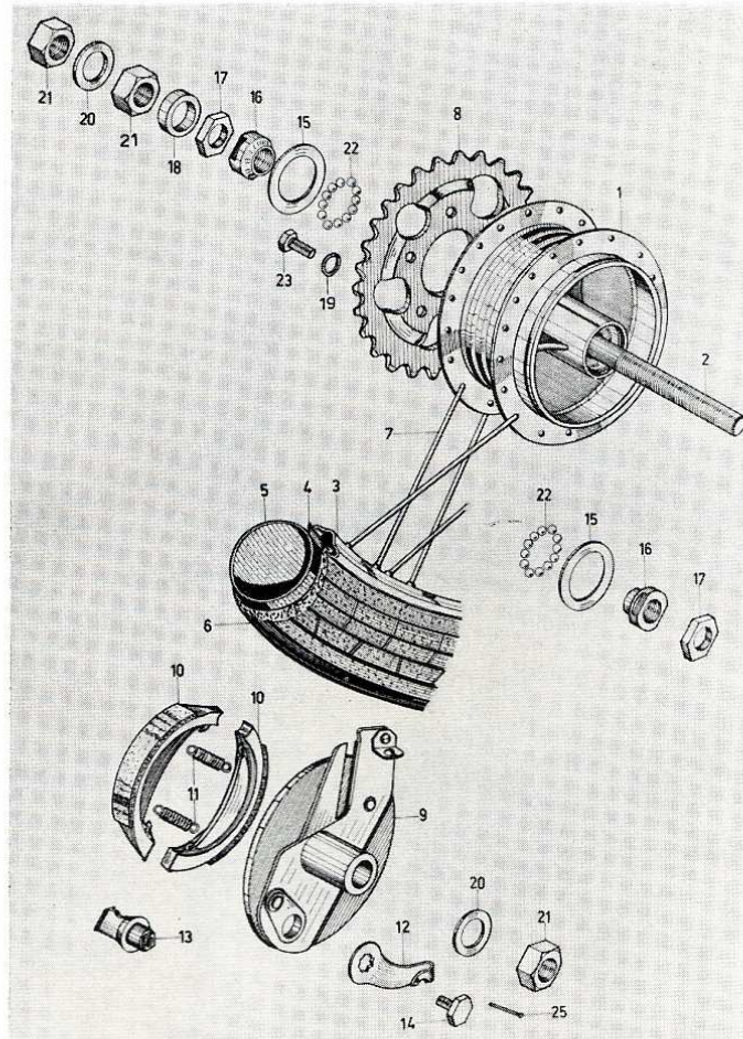
Fig. 31. — VUE ECLATEE DU MOYEU ARRIERE.
