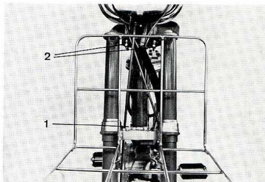
Fig. 6. — DEMONTAGE DU PORTE-BAGAGE.
