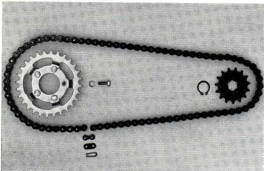
Fig. 28. — DEMONTAGE DE LA CHAINE.
